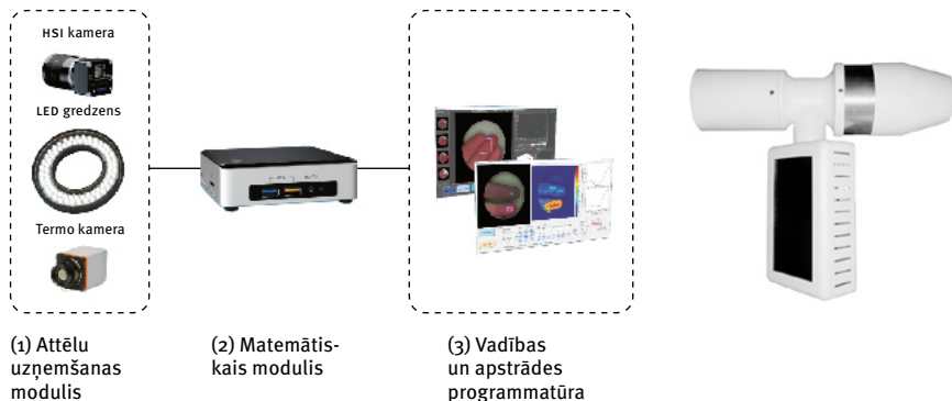
6. ATTĒLS. Sepses diagnostikas ierīces prototips; pa kreisi — sistēmas galvenās komponentes: termālā un hiperspektrālā kamera, pa labi — prototipa darba versija.
