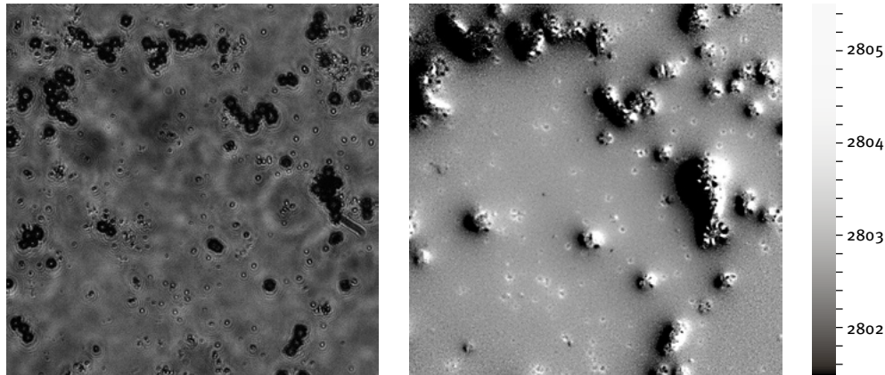
4. ATTĒLS. Attēla kreisajā pusē redzams optiskais attēls maisījumam no 2 \mu\text{m} un 0,5 \mu\text{m} diametra daļiņām, kas uzklāts piliena veidā, atļaujot tam nožūt ārēja magnētiskā lauka klātbūtnē. Attēla labajā pusē redzams šā paša reģiona magnētiskais attēls, kam blakus esošā krāsu kodu skala raksturo rezonanses mikroviļņu frekvences. Mērījumi veikti uz pārejas no m_s = 0 uz m_s = -1 .
