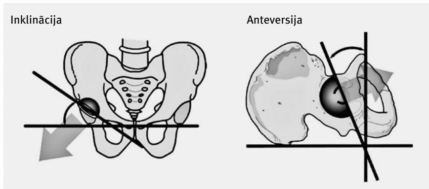
2. ATTĒLS. Acetabulārā komponenta inklinācija un anteversija. (Attēls ņemts no www.orthobullets.com )
