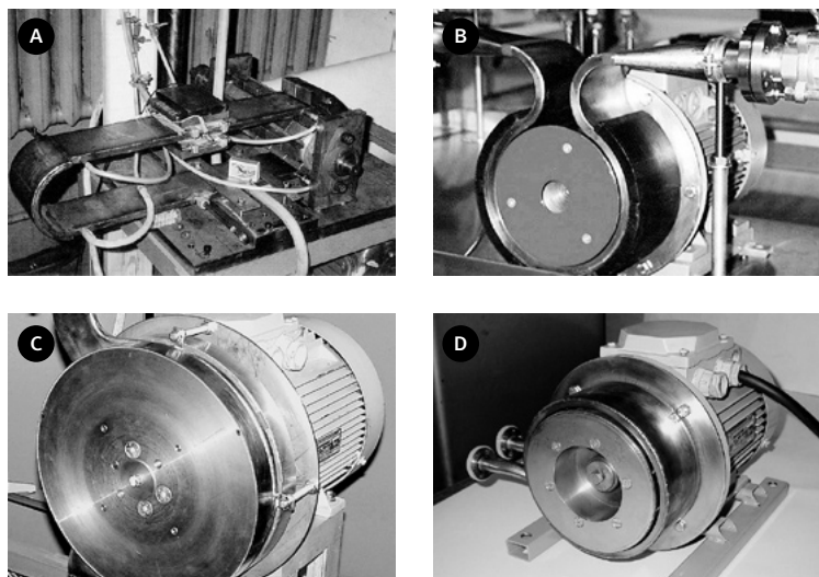
1. ATTĒLS. Pastāvīgo magnētu sūkņi: (A) pirmais realizētais pastāvīgo magnētu sūkņi; (B), (C), (D) pēc pasūtījuma LU Fizikas institūtā realizētie pastāvīgo magnētu sūkņi.
