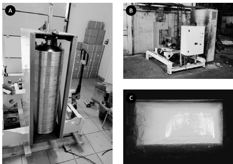
2. ATTĒLS. Industriāla izmēra rotējošu pastāvīgo magnētu maisītājs: (A) pastāvīgais magnēts ar 30 cm diametru; (B) rūpnīcā uzstādīts pastāvīgo magnētu maisītājs pie alumīnija krāsns; (C) krāsns iekšpuse ar izkausētu alumīniju.
