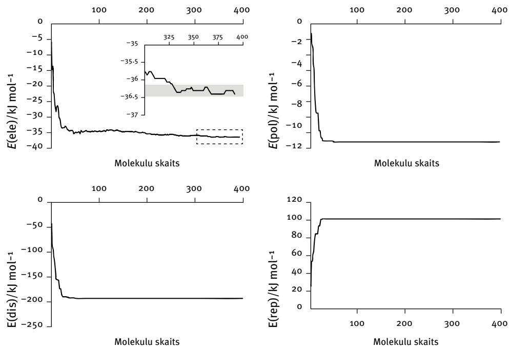
2. ATTĒLS. Kristālrežģa enerģijas (nenormētu) komponentu konverģence ( E(\text{ele}) – elektrostatiskā potenciāla enerģija; E(\text{pol}) – polarizācijas enerģija; E(\text{dis}) – dispersijas enerģija; E(\text{rep}) – atgrūšanās enerģija).
